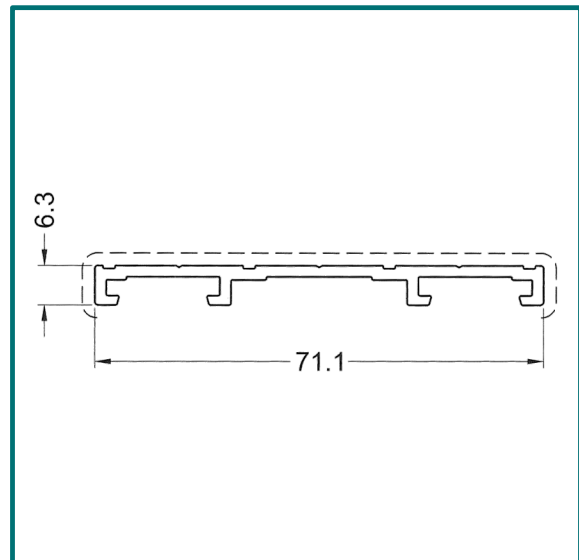
Seitlicher Rahmen 3-spurig
