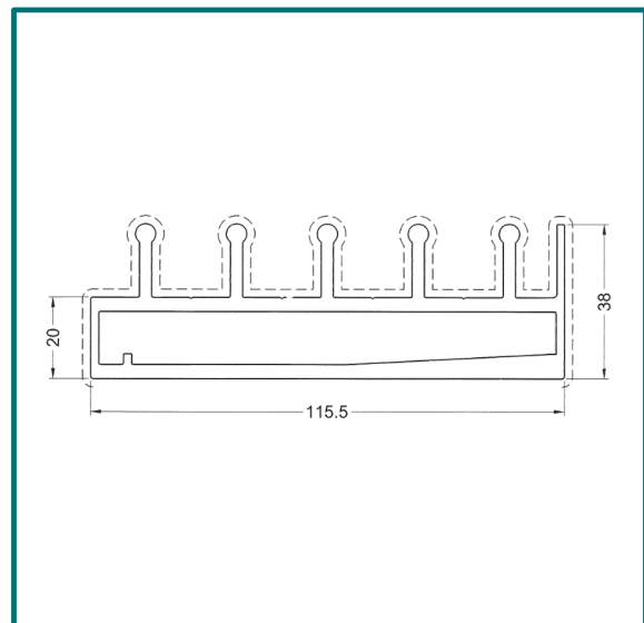
Untere Laufschiene 5-spurig
