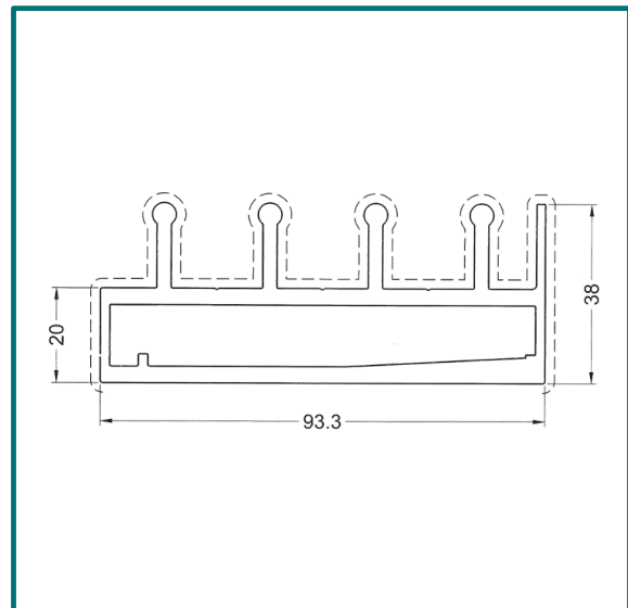
Untere Laufschiene 4-spurig
