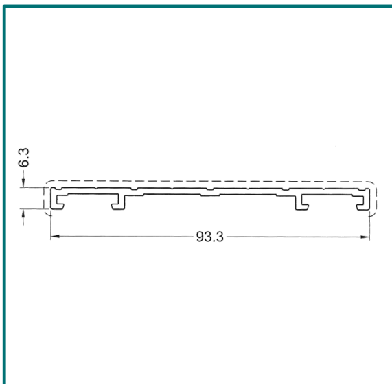
Seitlicher Rahmen 4-spurig
