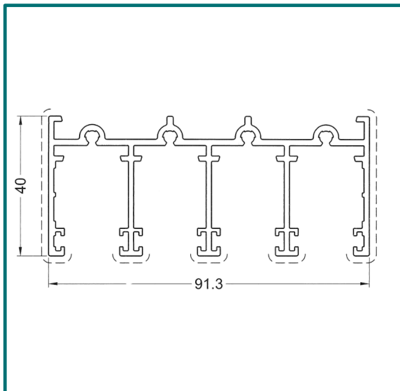
Obere Laufschiene 4-spurig
