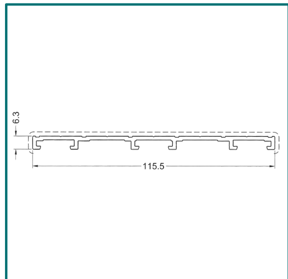
Seitlicher Rahmen 5-spurig
