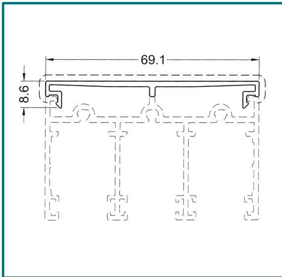
Obere Laufschiene 3-spurig mit Abdeckprofil
