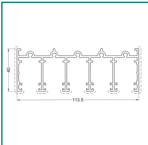
Obere Laufschiene 5-spurig
