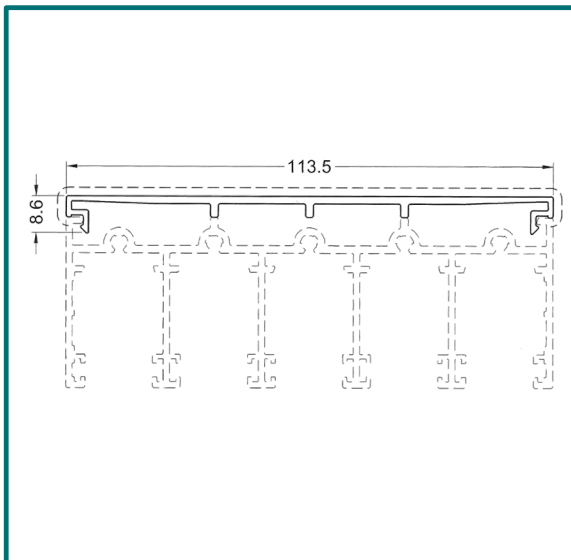
Obere Laufschiene 5-spurig mit Abdeckprofil
