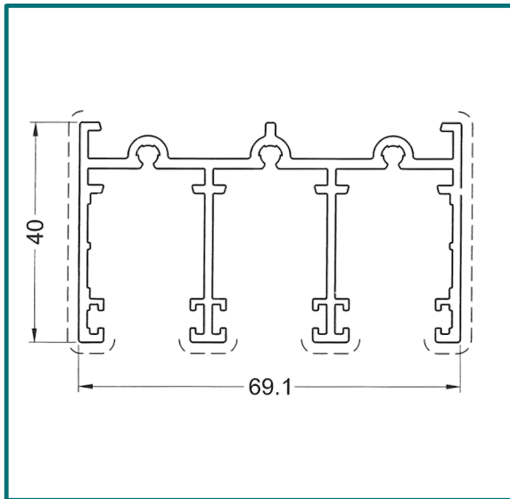
Obere Laufschiene 3-spurig
