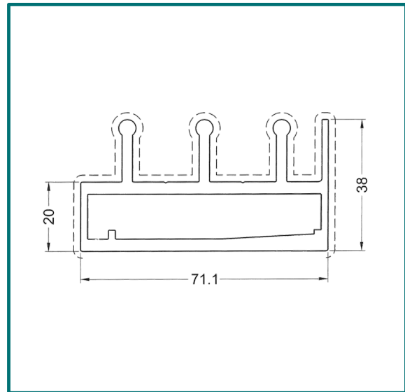
Untere Laufschiene 3-spurig
