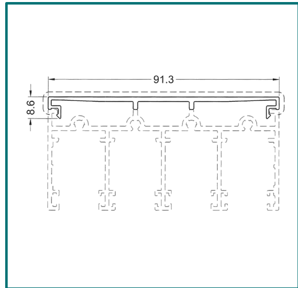
Obere Laufschiene 4-spurig mit Abdeckprofil
