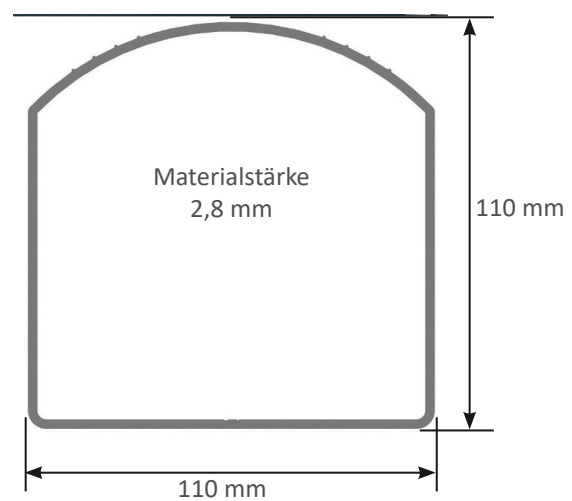
Pfostenprofil
